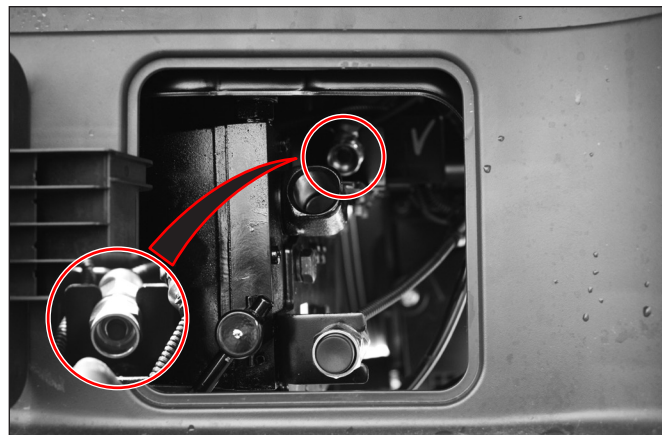
보조 시동 스위치
