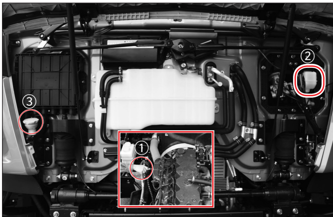
① 엔진오일 수준(캡탈핑 후 점검) ② 클리치액 수준 ③ 와셔액 수준
