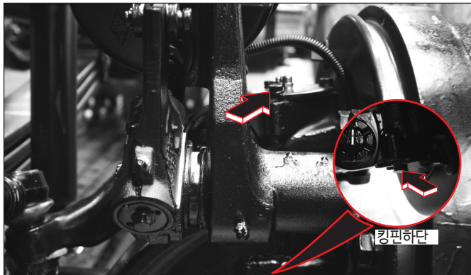
1) 킹핀
