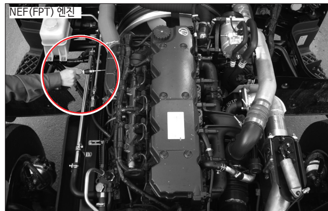
2) NEF(FPT) 엔진 : 캡을 올리면 엔진 왼쪽(운전석쪽) ECU 상단부에 게이지가 있습니다.
