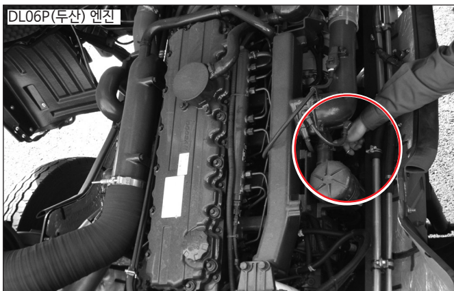
1) DL06P(두산) 엔진 : 캡을 올리면 엔진 오른쪽(조수석쪽) ECU와 오일 필터 사이에 게이지가 있습니다.
