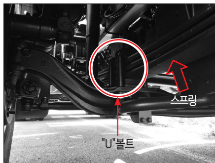
"U" 볼트
